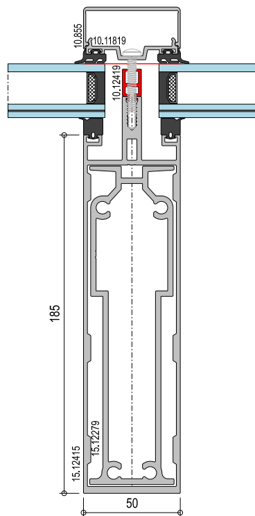
MR50 STIJL MET VERSTEVIGING
