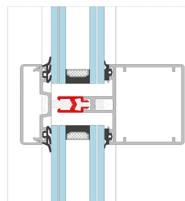
MR50 LIGGER VLAKKE AFDEKKAP
