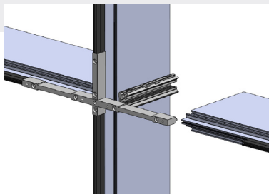
MR50 KRUIS VOOR AFSTEUNING GLAS
