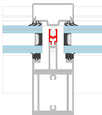
MR50 STIJL MET VERSTEVIGING
