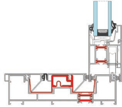
B45 TRI-SCHIENE
